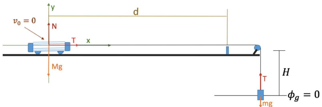
Figura 1. Esquema del carrito y sus fuerzas aplicadas.
