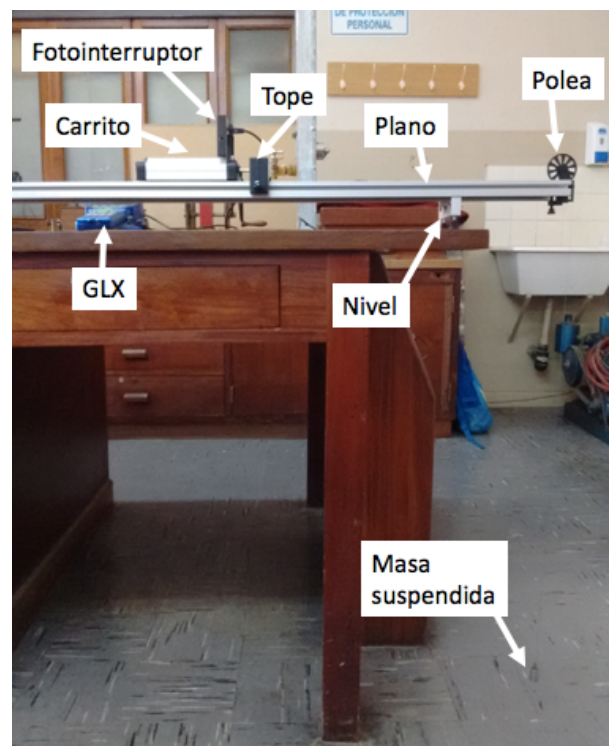
Figura 2. Montaje experimental
