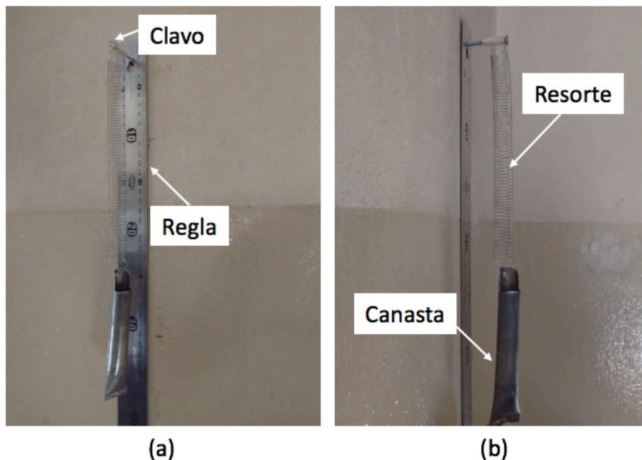
Figura 2. Foto de la representación esquemática del sistema para determinar la constante elástica. En (b) puede verse lateralmente la separación entre el resorte y la canasta y la pared.
