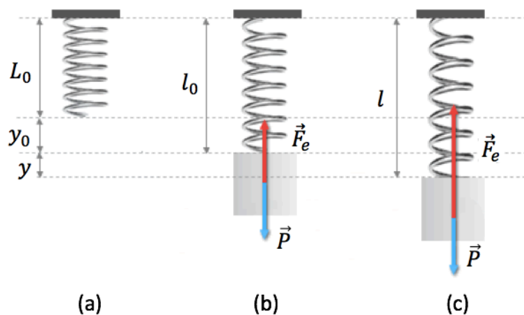
Figura 1. Representación esquemática de un cuerpo suspendido verticalmente del extremo de un resorte.
